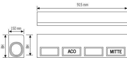
Dimensiones del elemento central para vado Dimensões do elemento central para rampa
